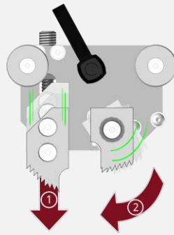
Griffes de serrage à double action (brevetées)
